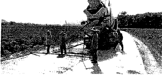
งานเทศคอนกรีต วันที่ 20 เม.ย. 2561 ณ ถนนสาย หนองกรับ - มาบหวายโสม พื้นที่หมู่ที่ 3 ต.หนองบัว อ.บ้านค่าย จ.ระยอง
